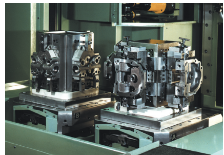
Wechselpaletten mit Aufspannwürfel Pallets with clamping column
