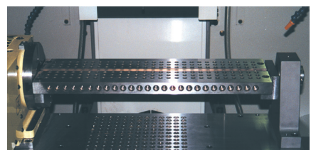
Spannbrücke mit Wiegenplatte Clamping bridge with central base plate
